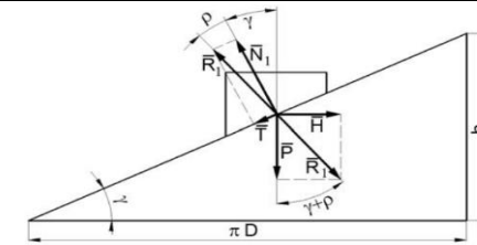
Rys. 2. Układ sił w gwincie śruby.
