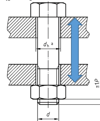
Rys. 3. Schemat badania połączenia śrubowego na rozciąganie.
